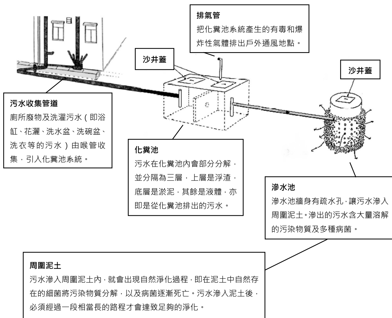
圖 1：化糞池和滲濾系統 ( 圖片由環保署提供 )
